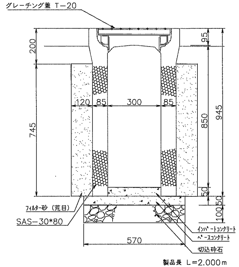
透水性門型側溝SAS-30*80 構造図 S=1/10 (消音タイプ)
