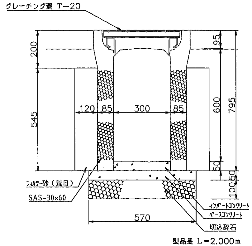
透水性門型側溝SAS-30*60 構造図 (消音タイプ) S=1/10
